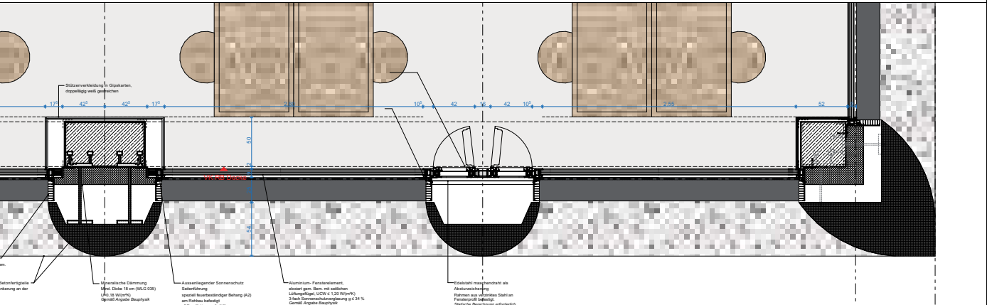
FASSADE
